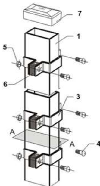
K Přichytka koncová
